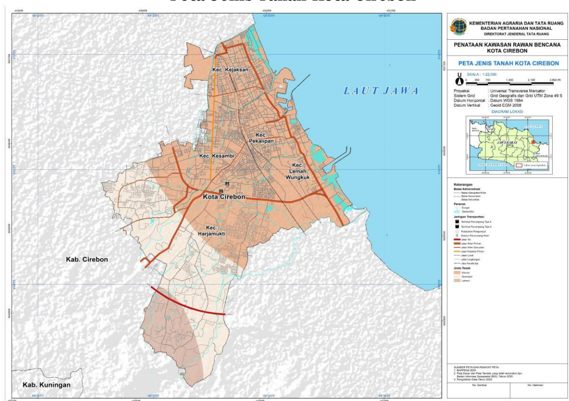
Gambar 2.4 Peta Jenis Tanah Kota Cirebon
