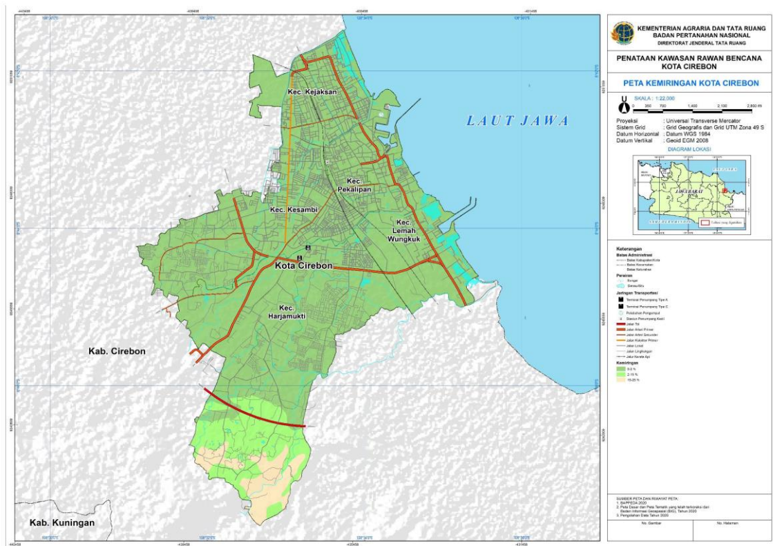
Gambar 2.3 Peta Kemiringan Lereng Kota Cirebon
